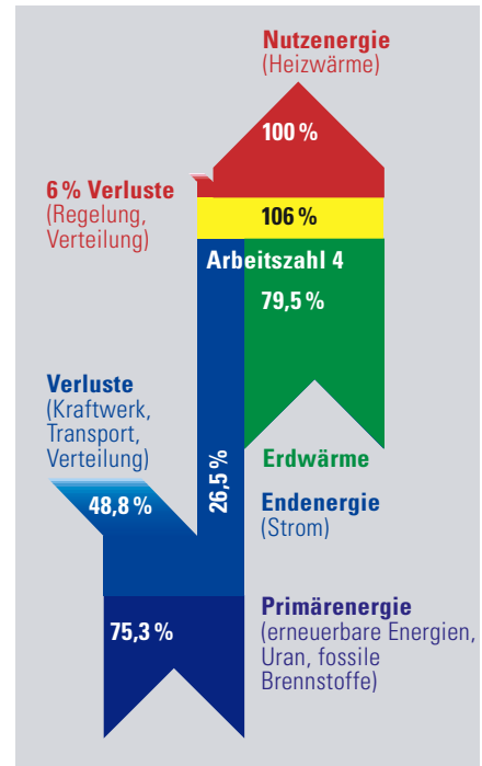
Energieflußdiagramm einer Erdwärmepumpen-Heizanlage mit einer Arbeitszahl von 4.
