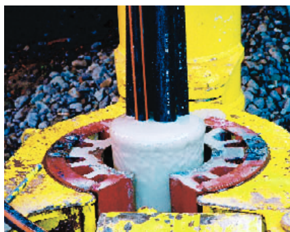
Zementation der eingebauten Doppel-U-Erdwärmesonde.
